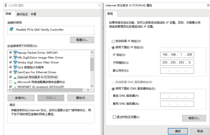
图 2-3 PC 网卡配置
