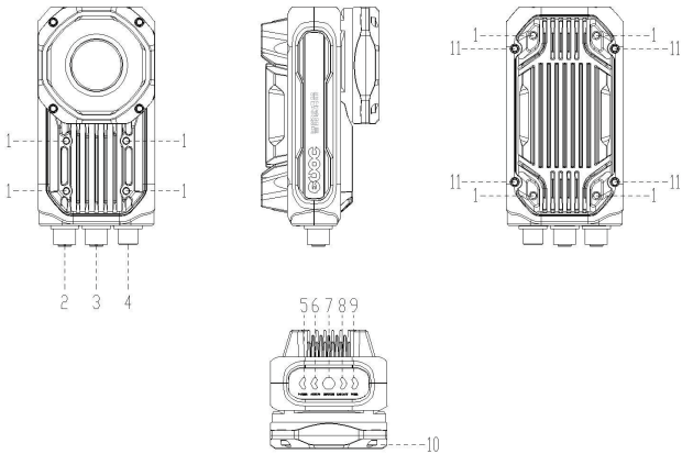
图 1-1-2 R-5000 设备外观
